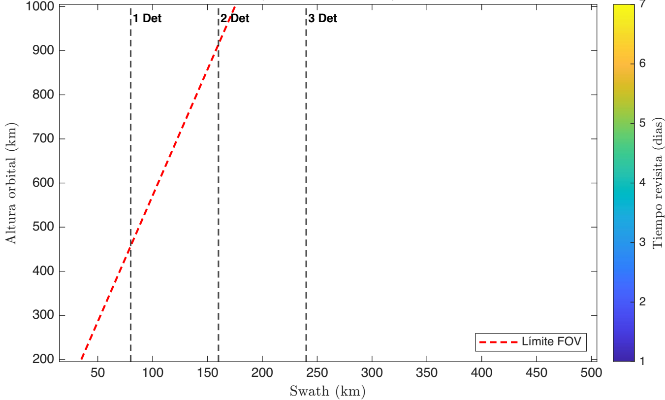
Tiempo Revisita - 2 Satelite(s); 1 Telescopio(s): Refractivo; Detector 3 (Blanco: \geq 7 dias)
